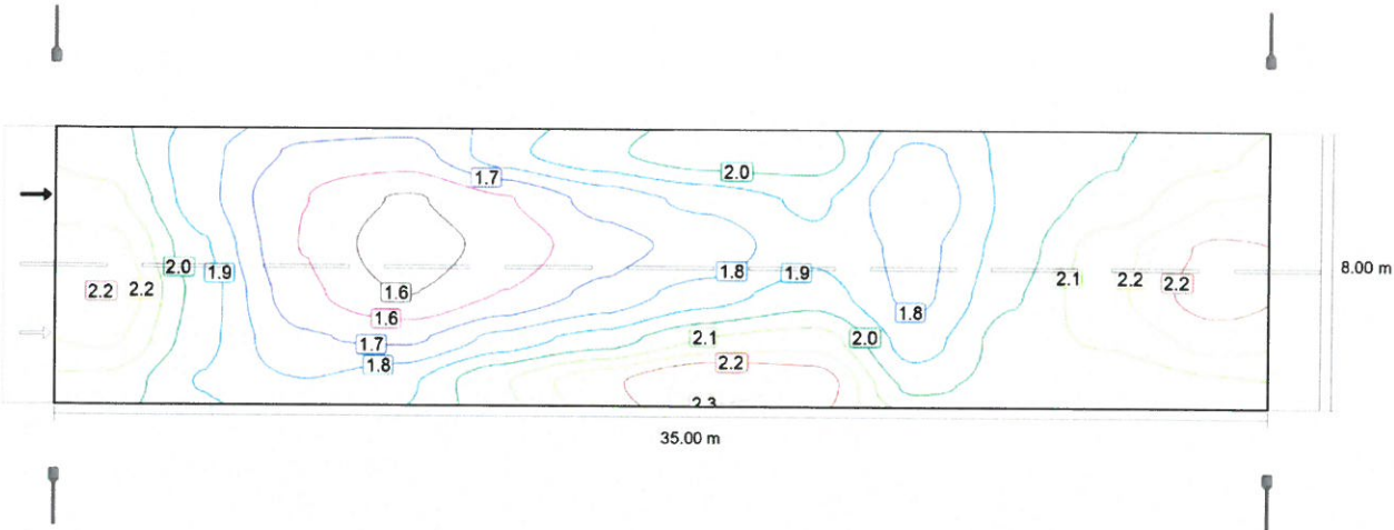
Observator 2: Densitatea luminii la instalația nouă [cd/m²] (Linii Isolux)
