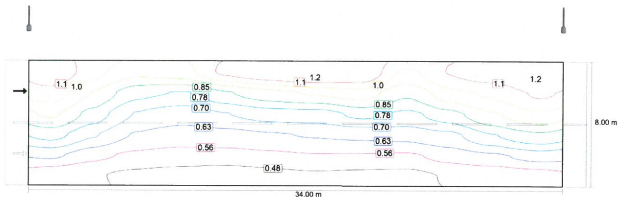
Observator 2: Valoarea de întreținere, densitatea luminii cu carosabil uscat [ \text{cd/m}^2 ] (Linii Isolux)
