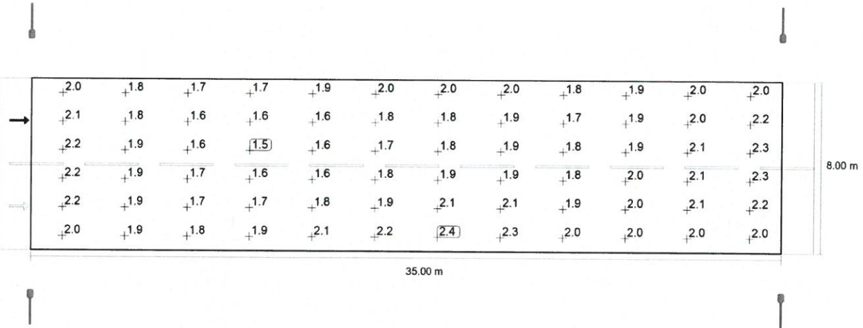
Observator 2: Densitatea luminii la instalația nouă [cd/m²] (Raster valoric)
