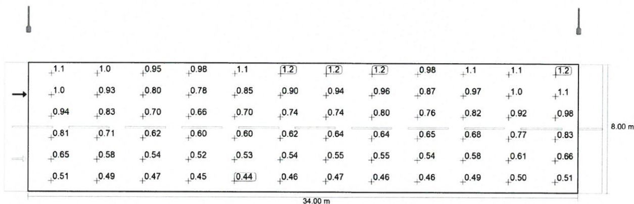
Observator 2: Valoarea de întreținere, densitatea luminii cu carosabil uscat [ \text{cd/m}^2 ] (Raster valoric)
