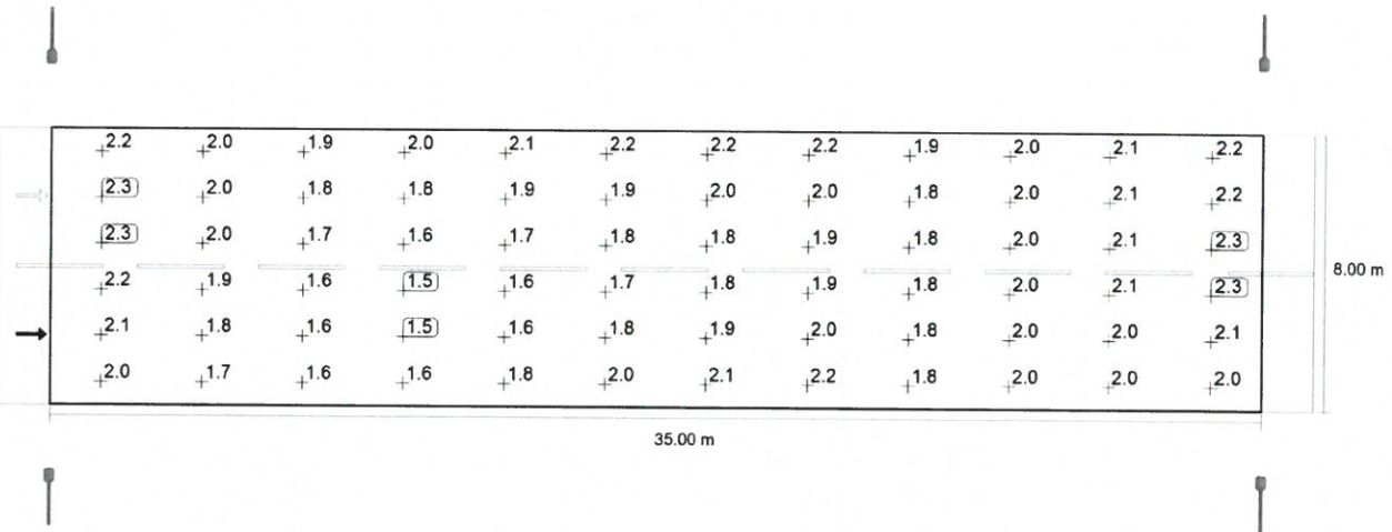
Observator 1: Densitatea luminii la instalația nouă [cd/m²] (Raster valoric)
